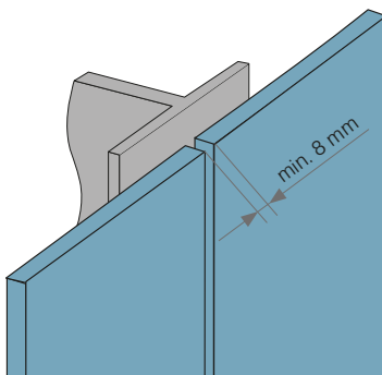
Abb. a. Offenes Fugensystem
